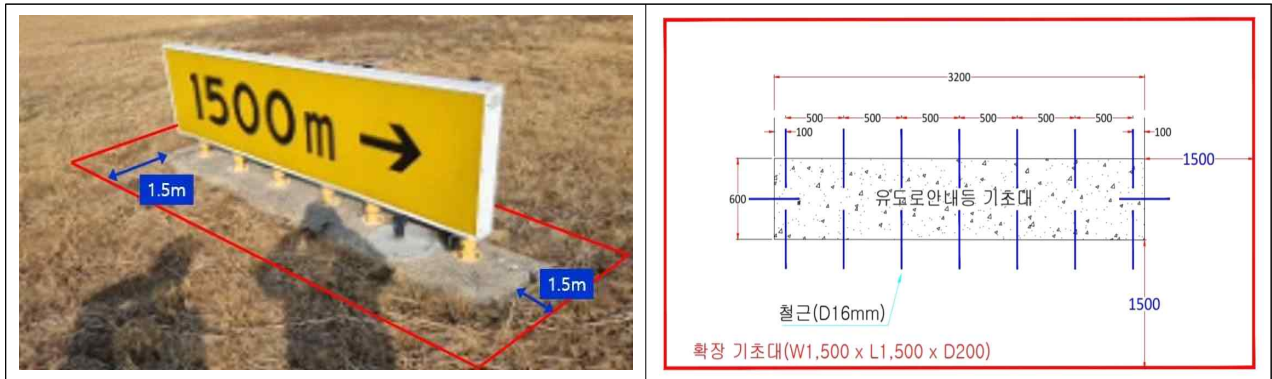
【그림1】 기초대 확장 평면도(예시)
