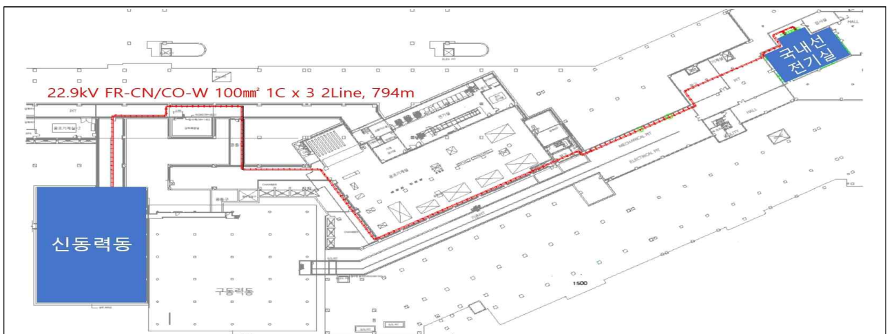
【그림1】 국내선 전기실 전원 선로 포설 계획(신동력동 ~ 국내선 전기실)
