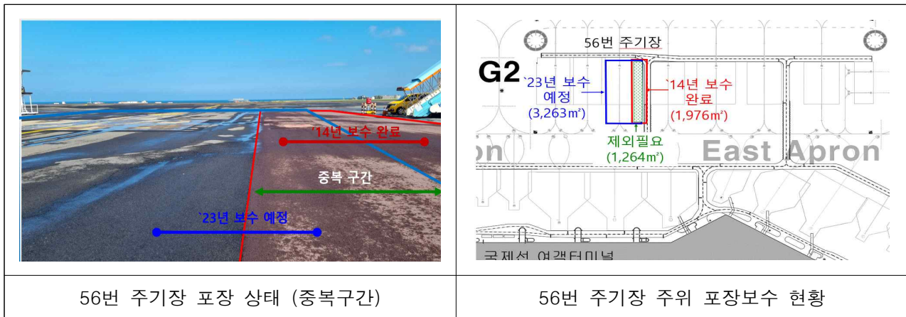
【그림】 56번 주기장 주변 포장 상태 및 보수현황
