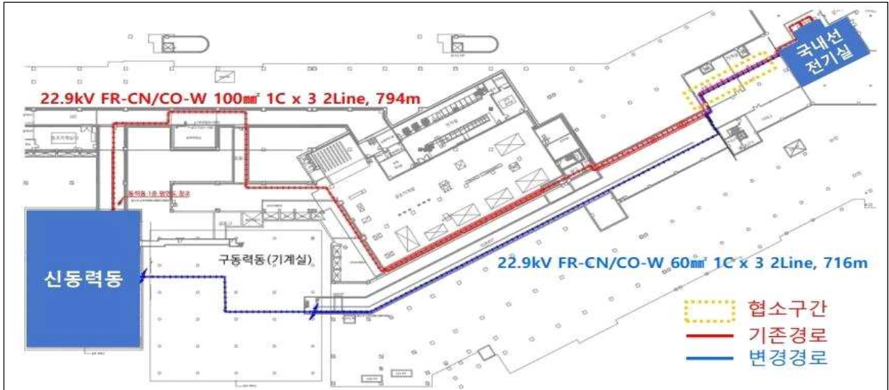
【그림3】 기존 고압인입선로 재사용 구간(신동력동 ~ 국내선 전기실)
