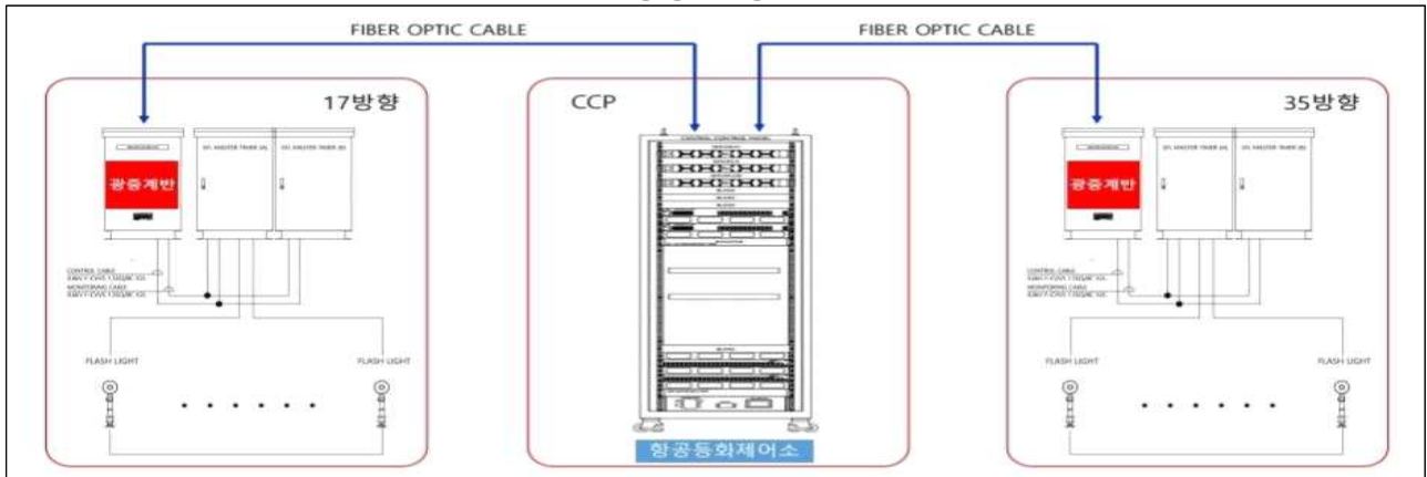
【그림2】 섬광등용 광중계반 구성도
