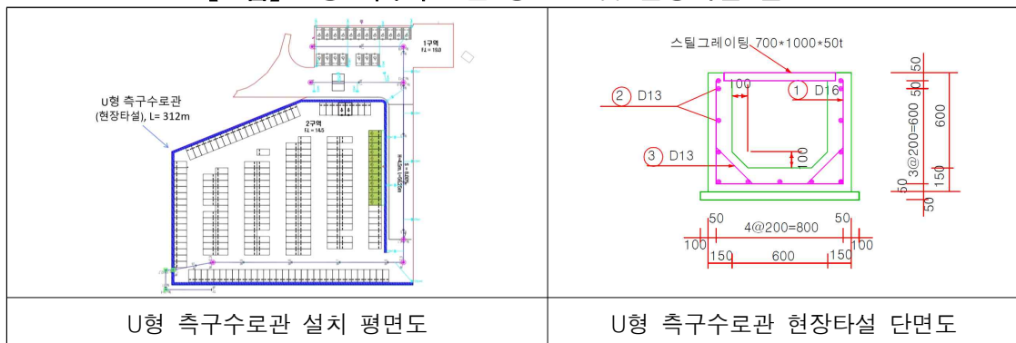
【그림】 U형 측구수로관 평면도 및 현장타설 단면도
